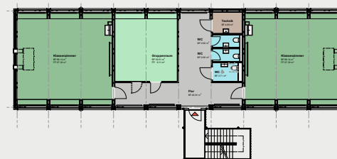
Plan d'étage 10 modules forment 1 étage
