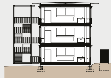
Exemple de coupe transversale d'un bâtiment de trois niveaux
